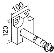
Uchwyty ścienny z lewej
