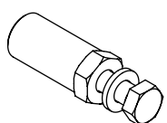
Redukcja M 16 → M 12 / SW 27 50 mm
