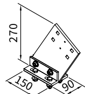
Uchwyt krokwiowy wysokość płaskownika 270 mm
