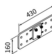
Płyta mocująca A 430 × 160 × 12 mm
