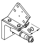
Uchwyt krokwiowy wysokość płaskownika 150 mm prawy
