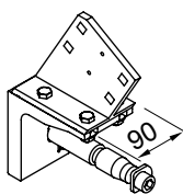
Uchwyt krokwiowy wysokość płaskownika 150 mm prawy
