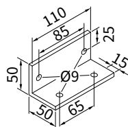
Kątownik mocujący
