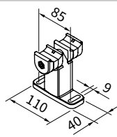
Podwójny uchwyt szynowy u góry ruchomy
