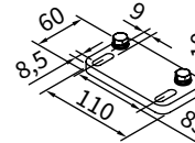
Płyta adaptera do uchwyty szynowego 110 × 60 × 10 mm
