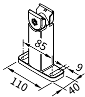
Uchwyt szynowy u góry ruchomy
