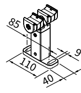
Podwójny uchwyt szynowy u góry ruchomy
