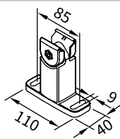
Uchwyt szynowy u góry ruchomy
