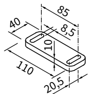
Płyta dystansowa do uchwyty szynowego 110 × 40 × 10 mm
