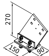
Uchwyt krokwiowy nakładka 270 mm
