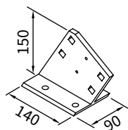
Uchwyty krokwiowy nakładka 150 mm
