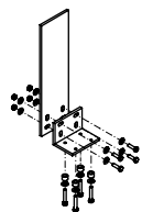
Nakładka i kątownik do montażu krokwiowego
