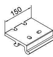
Uchwyty stropowy 150 mm
