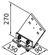
Uchwyty krokwiowy nakładka 270 mm
