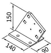
Uchwyt krokwiowy nakładka 150 mm
