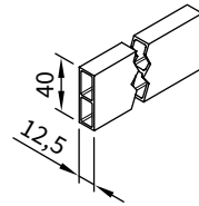
Listwa dystansowa do profilu ochronnego mocowanego do ściany Długość
