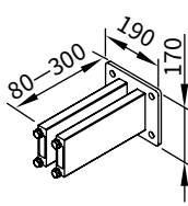
Uchwyt dystansowy do konsoli ściennej 70867.
