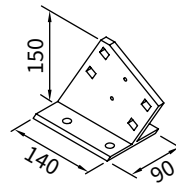
Konsola krokwiowa Nakładka 150 mm
