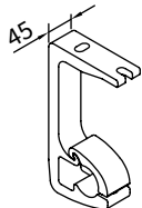
Konsola stropowa dodatkowa konsola przy 3 ramionach przegu- bowych
