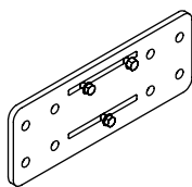
Płyta mocująca A Ściana 160 × 430 × 12 mm
