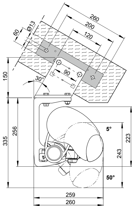
z konsolą krokwiową 150 mm (71612.)
