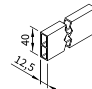
Listwa dystansowa do profilu ochronnego mocowanego do ściany
