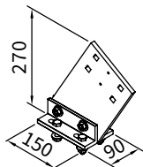
Konsola krokwiowa Nakładka 270 mm patrz krokwie- mocowanie z dodatkową nakładką"
