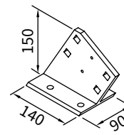
Konsola krokwiowa Nakładka 150 mm
