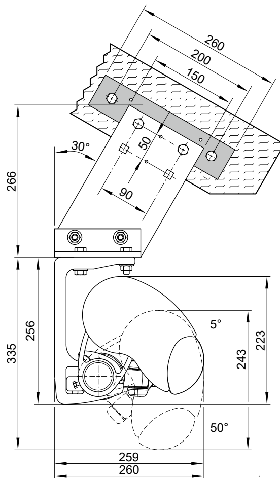
z konsolą krokwiową 270 mm (71659.)
