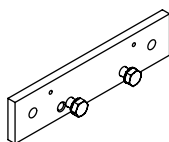
Dodatkowa nakładka Krokwie 260 x 60 x 12 mm
